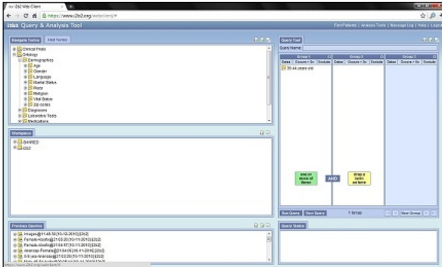
Actual Screenshot of i2b2 Web Client
